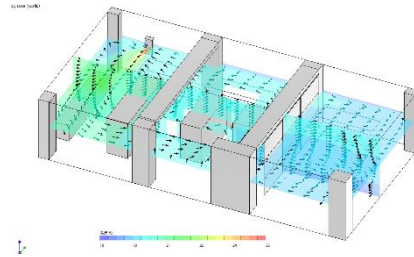
気流制御(空気循環)
