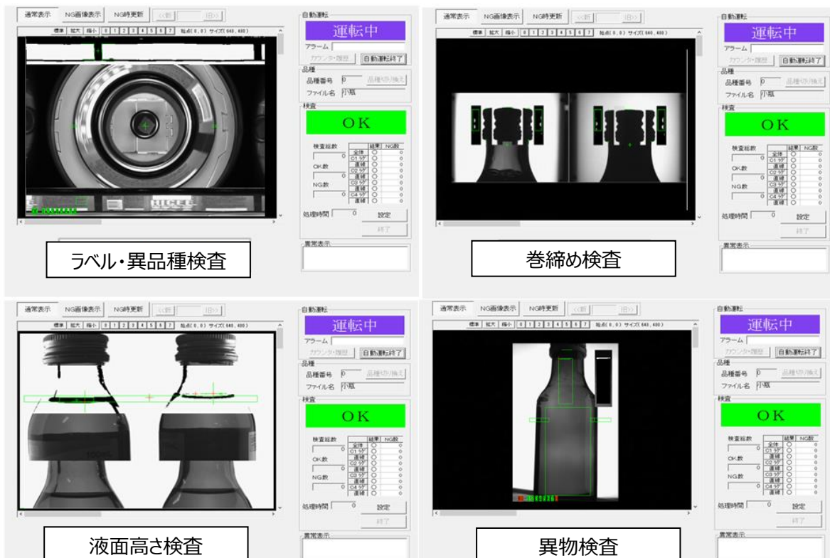
「検査画面」
