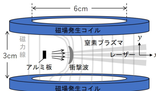
図2. 実験概略図
