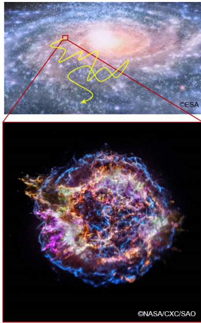
図4. 上：天の川銀河と宇宙線軌道（黄色線）の想像図 下：超新星残骸（Cas A）
