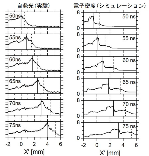
図5. 左：実験により、プラズマからの発光で捉えた衝撃波の形成過程。発光強度のピーク位置（縦実線）が時間とともに移動。ピークの前面（右側）にフット ※3 が形成されており、その空間サイズが時間とともに変化している。
