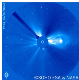
図1. 太陽面爆発に伴って宇宙空間を伝播する衝撃波 (ESA/NASA 提供)
