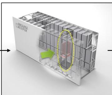
⑤移載機が荷物の入ったボックスを搬送
