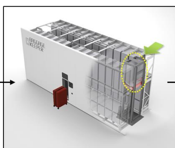
② 移載機が荷物を入れるボックスを棚からピックアップ
