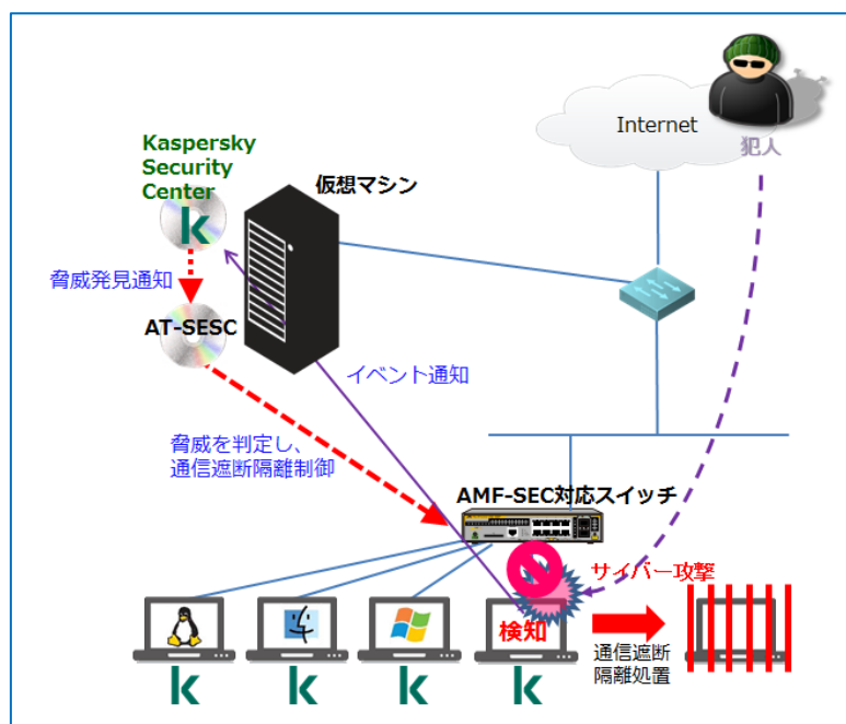
図：システム連携構成概要
