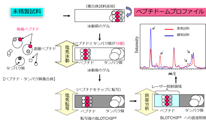
図3 BLOTCHIP®-MS法
