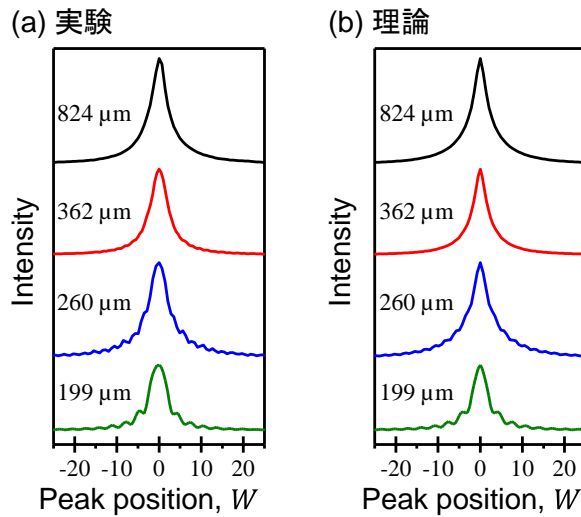
図 3 (a) ロッキングカーブ測定により得られた回折強度の振動曲線 (PF BL-20B で測定) (b) 動力的回折理論より予測される理論曲線 結晶の厚さを変化させると、観測される振動の間隔が変化する。
