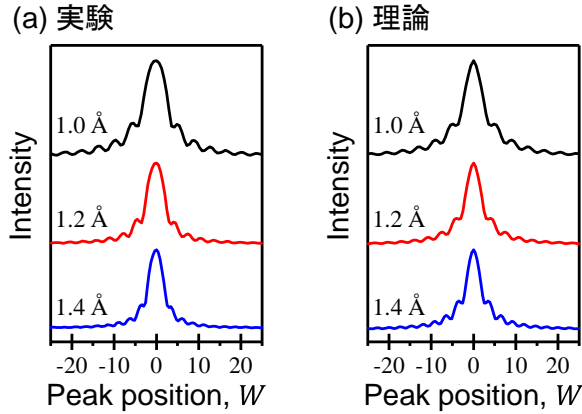
図 2 (a) ロッキングカーブ測定により得られた回折強度の振動曲線 (PF BL-20B で測定) (b) 動力的回折理論より予測される理論曲線 入射 X 線の波長を変化させると、観測される振動の間隔が変化する。
