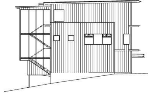
南立面图
