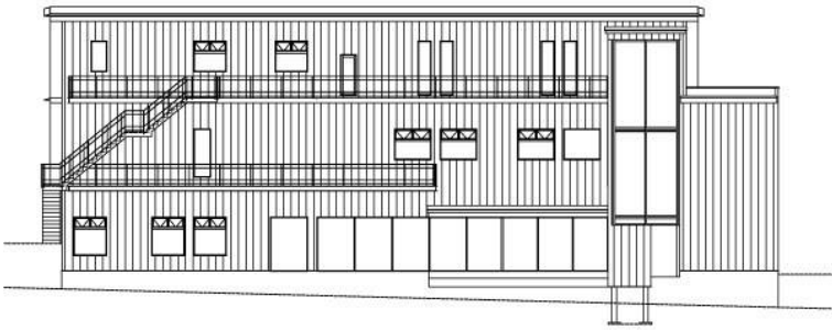
西立面图
