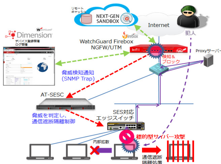
図：SES と Firebox シリーズとの連携構成概要
