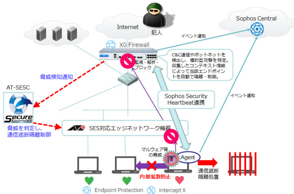
<図 : SES と Sophos XG Firewall 連携構成概要>
