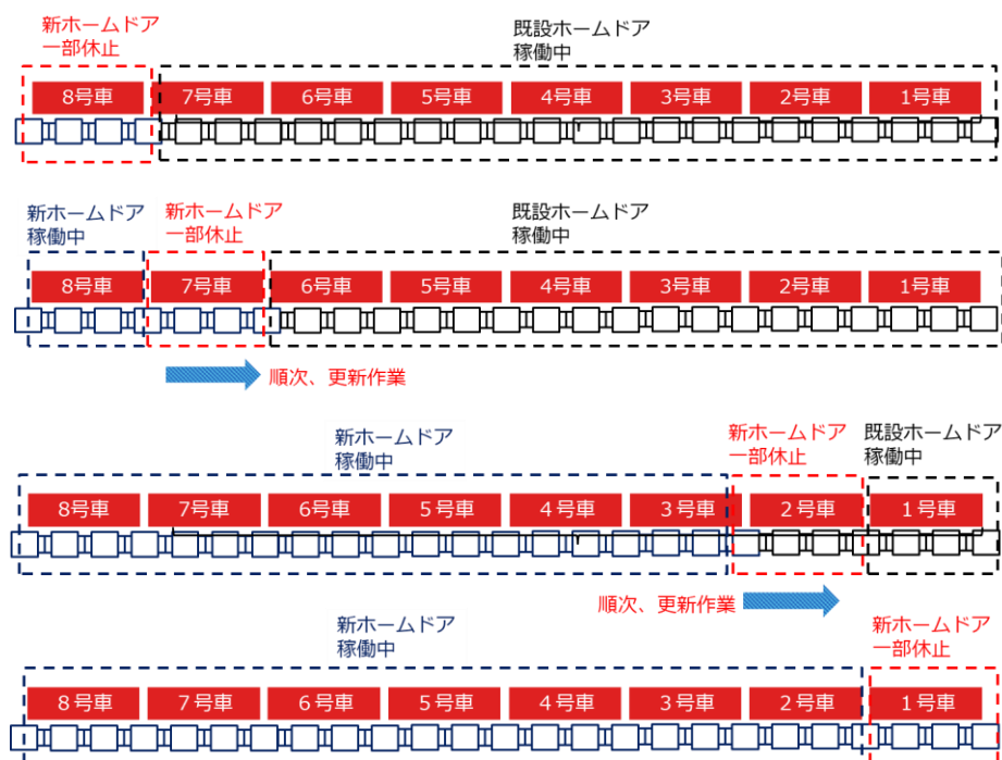
更新工事 概略図
