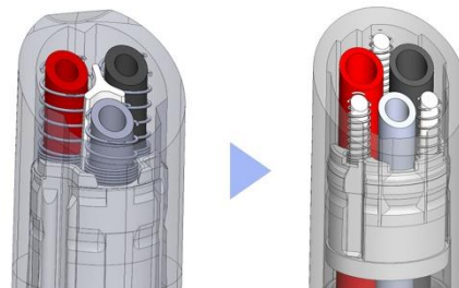
▲サイドスプリング機構イメージ
