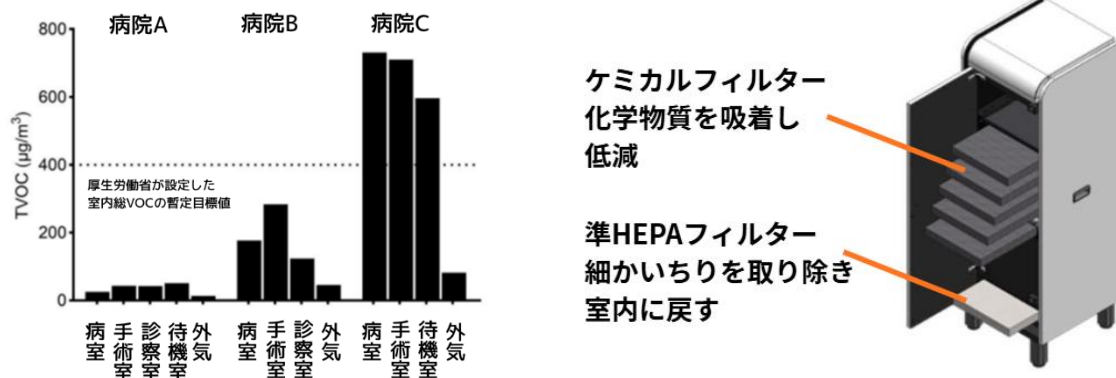
左: VOC 低減型空気清浄機稼働・未稼働時の室内の総 VOC (動物病院 A、動物病院 B は VOC 低減型空気清浄機を稼働。動物病院 C は未稼働。) 右: 開発した VOC 低減型空気清浄機の内部構造
