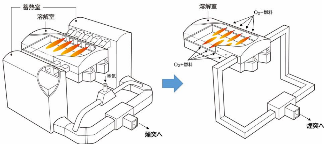
従来の燃焼方式（左）、酸素燃焼方式（右）
